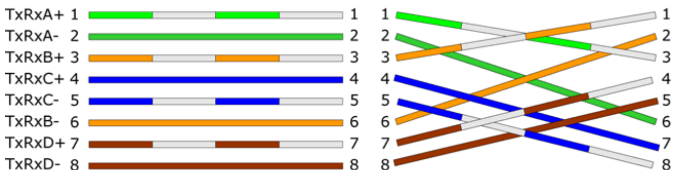
Patchkabel 1:1
